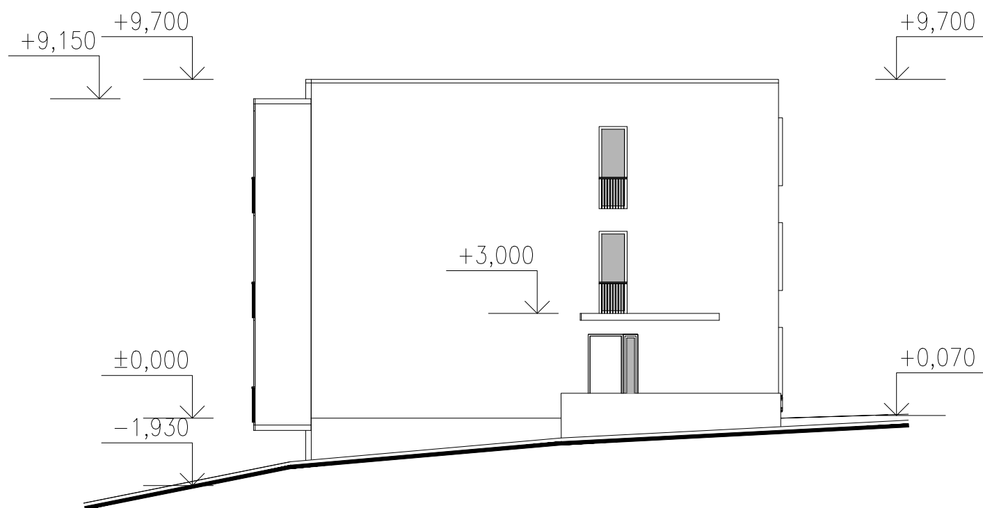
POHĽAD SEVEROVÝCHODNÝ
