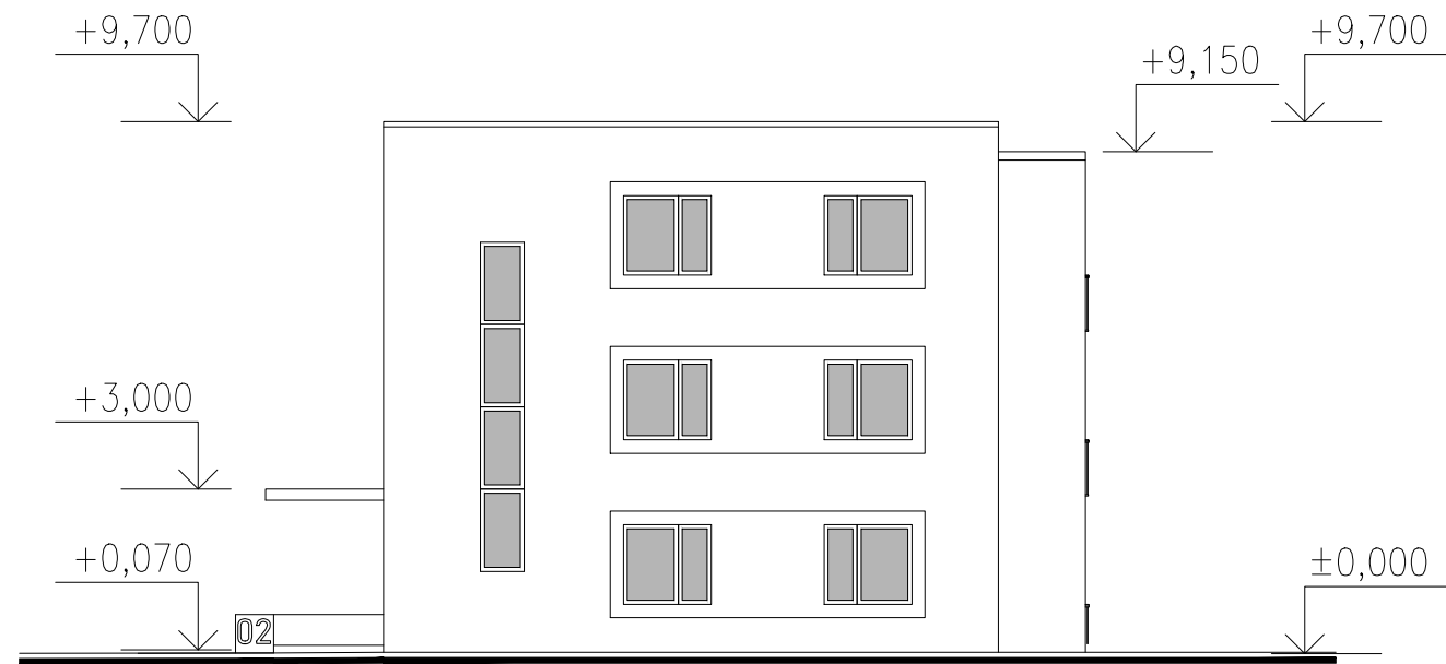
POHĽAD SEVEROZÁPADNÝ
